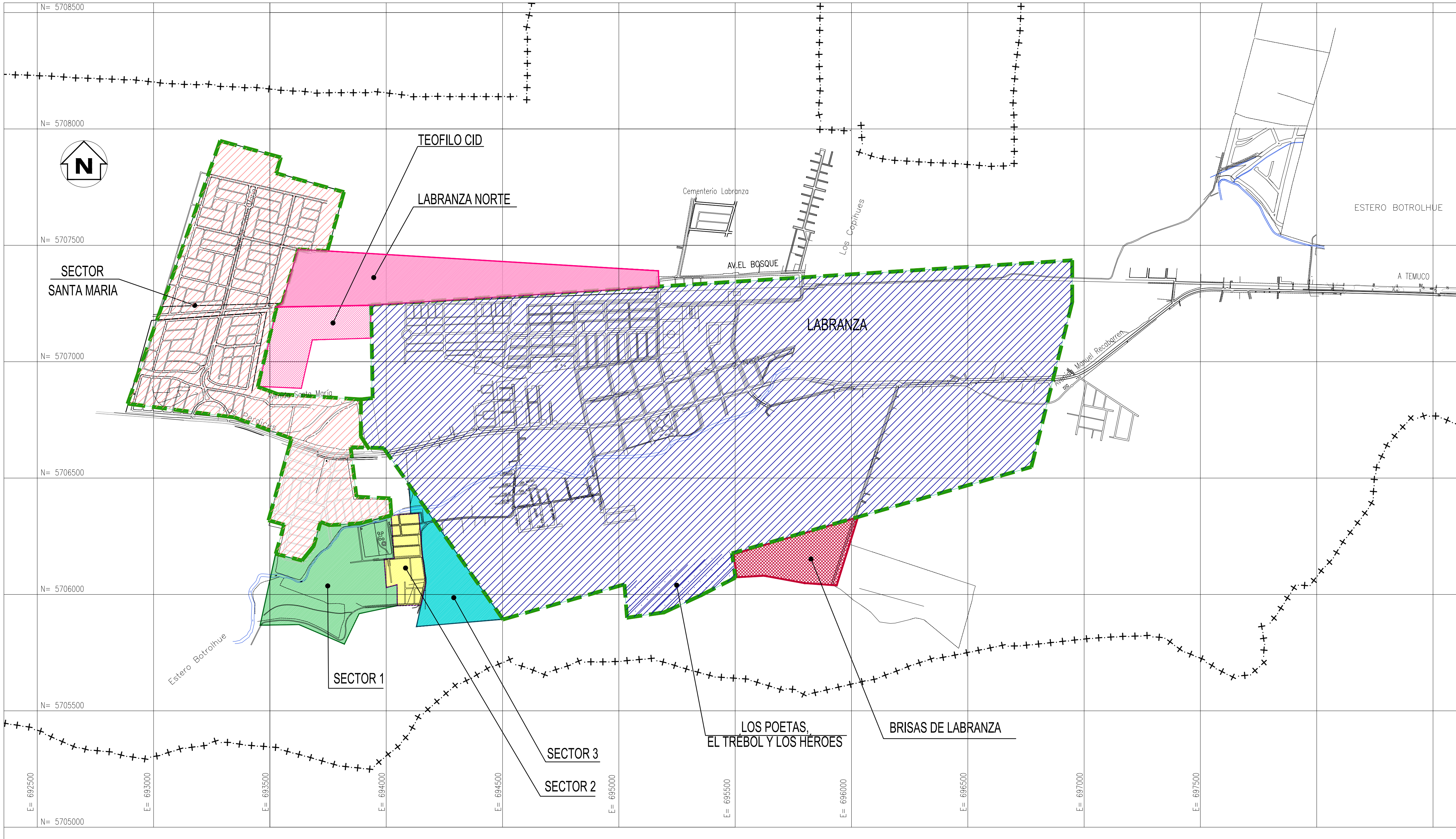
PLANTA GENERAL LABRANZA ESCALA 1 : 10.000
