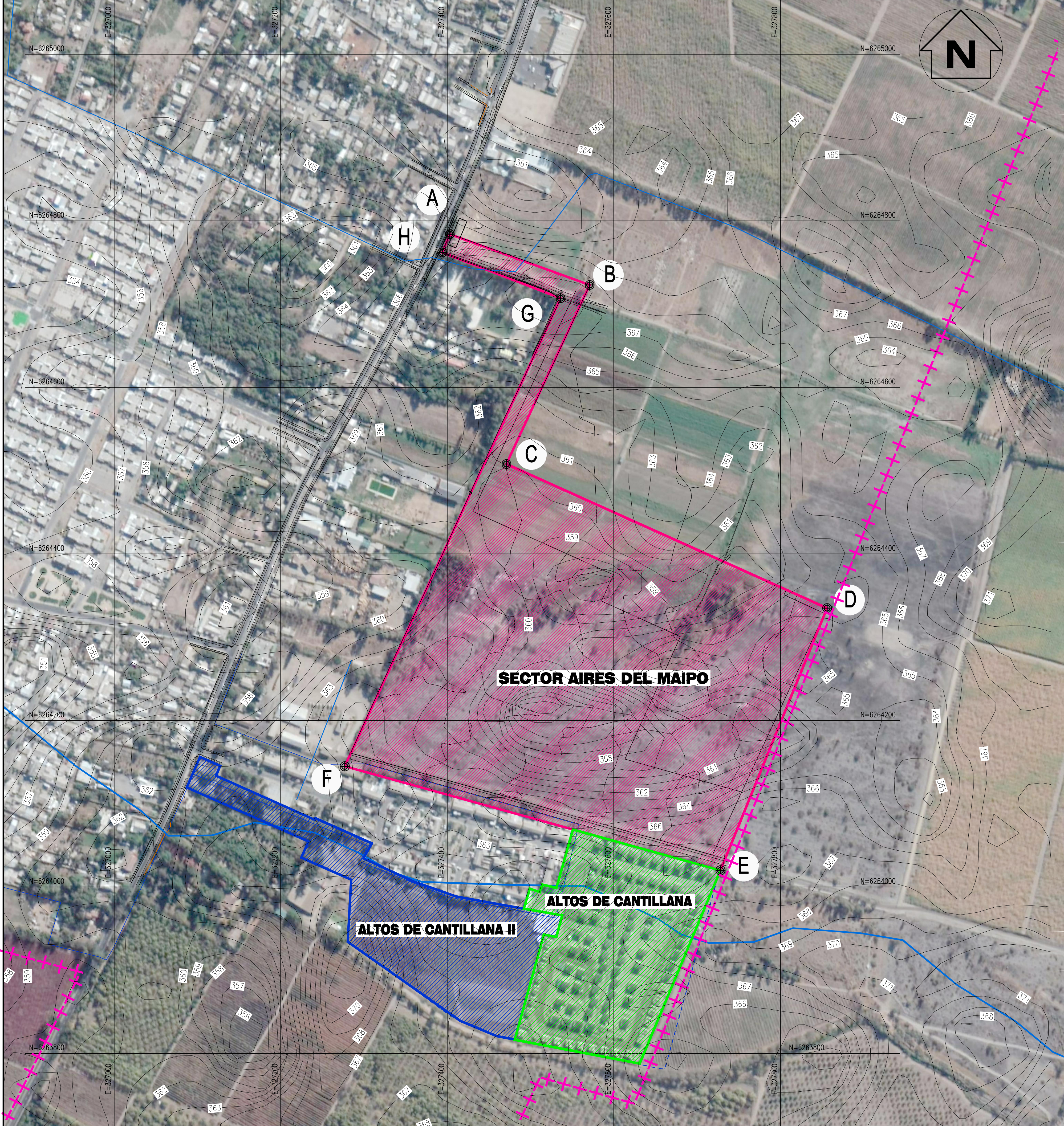
PLANTA GENERAL ESCALA 1: 2.500
